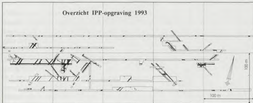
Gegraven proefsleuven in de Abtswoudse Polder en de daarin aangetroffen percelingsgreppels. Tekening: IPP.
