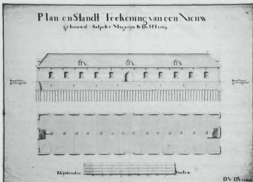
I. D. van der Velden maakte deze tekening van het aanzicht en de plattegrond van het, volgens zijn aangave, in 1769 gebouwde salpetermagazijn (GAD).
