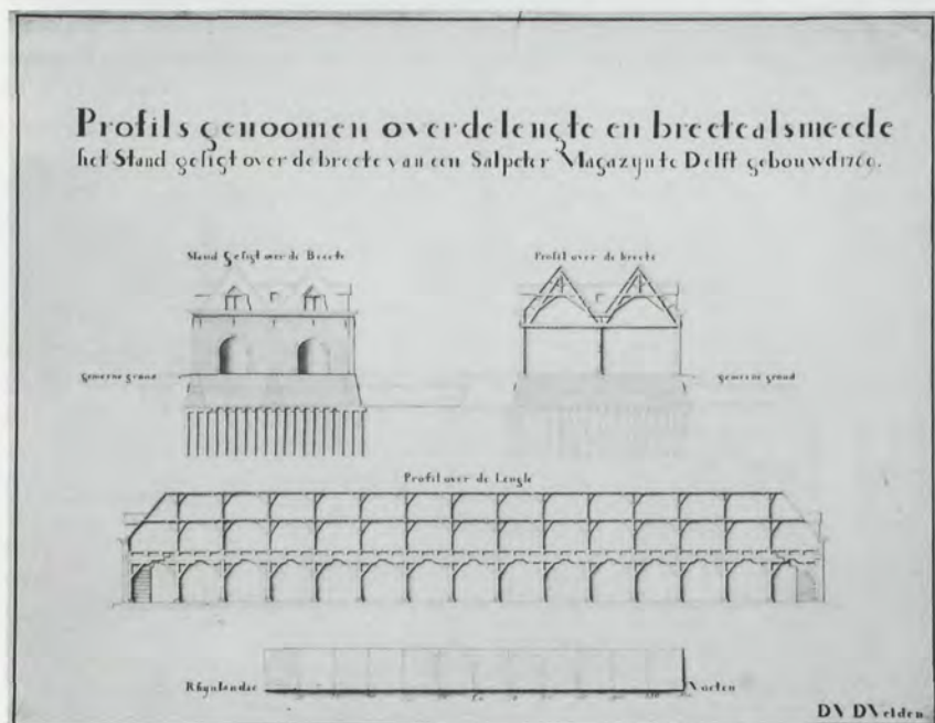
2. Een tekenaar met de initialen I.D. tekende onder meer een kopgevel en een dwarsdoorsnede. De tweebeukige opzet is goed te zien (GAD).
